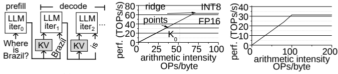
Fig. 1. An LLM autoregressive inference.
